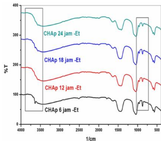
Gambar 4. Spektrum FTIR CHAp dari Goniopora cuci etanol dengan waktu sonikasi 6 jam sampai dengan 24 jam
