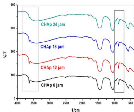
Gambar 3. Spektrum FTIR CHAp dengan waktu sonikasi 6 jam sampai dengan 24 jam
