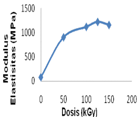
Gambar 8. Hubungan dosis radiasi terhadap modulus elastisitas
