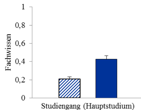
Abb.4: Fachwissen
