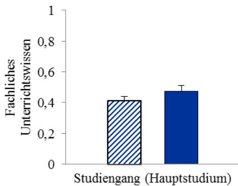
Abb.5: Fachliches Unterrichtswissen
