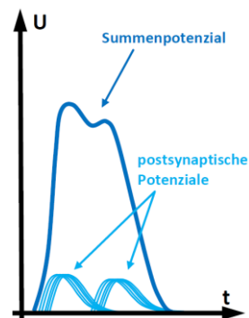
Abb. 2: Skizzenhafte Überlagerung postsynaptischer Potenziale zu einem starken Summenpotenzial im Kortex.
