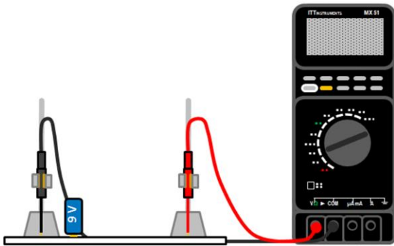
Abb. 5: Aufbau eines Analogieexperimentes zum Dipolmodell der EEG-Entstehung; die Schüler/innen positionieren 9V-Blockbatterien (Modelldipole) geometrisch unterschiedlich zu fest positionierten Messelektroden und protokollieren die dabei an einem Voltmeter gemessenen Gleichspannungen.
