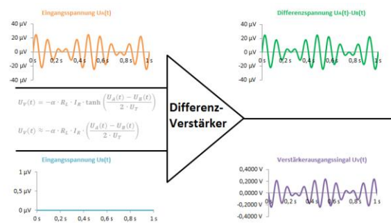
Abb. 7: Beispiel des Ausgabebildschirms der Simulation einer Referenzableitung; allgemein lassen sich in der Computersimulation die Amplituden, Frequenzen und Modulationen der Eingangssignale sowie die Parameter des Differenzverstärkers sowohl durch direkte Eingabe, wie auch durch Verwenden vorgefertigter Schieberegler verschieden einstellen, wobei sich der Ausgabebildschirm interaktiv an die momentane Einstellung anpasst. Hierdurch lassen sich unterschiedliche Szenarien leicht simulieren.
