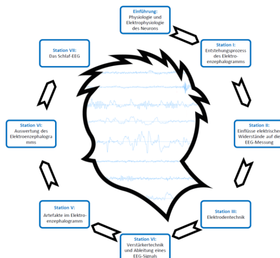
Abb. 4: Ablauf des Schülerforschungstages als Makrostruktur; die Schüler/innen erarbeiten an acht in ihrer Reihenfolge festen Etappen zentrale Aspekte des EEGs mit dem Ziel die Grundprinzipien der Elektroenzephalographie als ein facettenreiches Gesamtes darzustellen.
