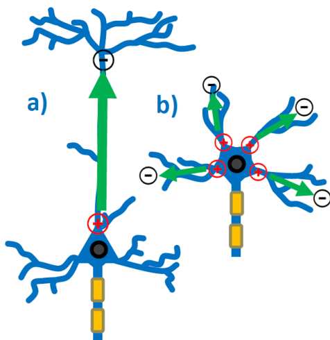
Abb. 3: Veranschaulichung kortikaler Dipole an den Dornfortsätzen von Pyramiden- (a) und Sternzellen (b); zu beachten ist, dass die Richtung der Dipolvektoren üblicherweise genau entgegen der in der klassischen Physik üblichen gewählt ist.
