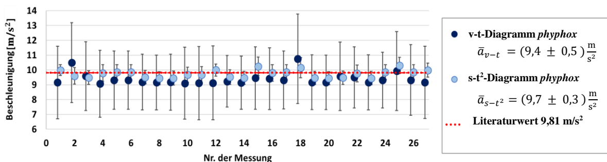
Abbildung 9: Ergebnisse von 27 Messungen zur Bestimmung der Erdbeschleunigung. Aufgetragen sind die bestimmten Beschleunigungswerte mit ihren Unsicherheitsintervallen. Sortiert nach Auswertungsmethoden: Geschwindigkeits-Zeit-Diagramm (dunkelblau), Weg-Zeit 2 -Diagramm (hellblau) und der theoretische Wert (rot). Ebenso sind die Mittelwerte mit den Standardabweichungen zu den beiden Auswerteverfahren angegeben.
