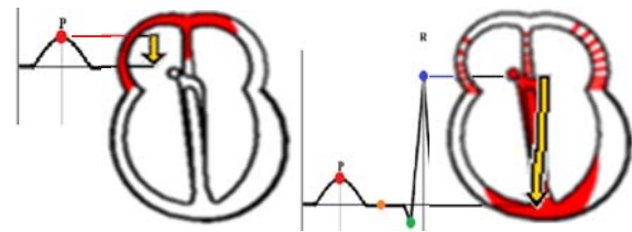
Abbildung 5: Entstehung einer EKG-Kurve
