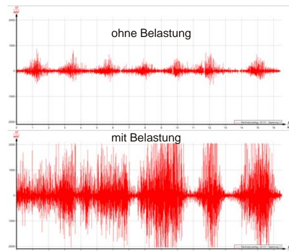
Abbildung 10: aufgenommene Elektromyogramme
