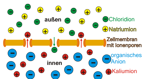
Abbildung 1: Ladungstrennung bei einer Zelle (nach [2])
