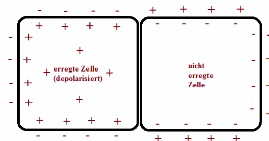
Abbildung 2: Außenräume der Zellen
