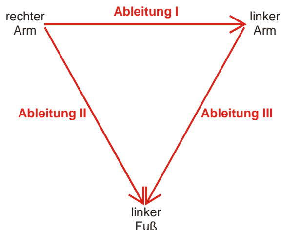
Abbildung 4: Das Einthoven-Dreieck
