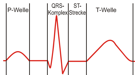
Abbildung 6: charakteristische EKG-Kurve
