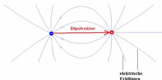
Abbildung 3: Entstehung des Dipols
