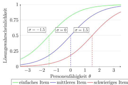
Abb. 2: Theoretischer Verlauf der Itemfunktion
