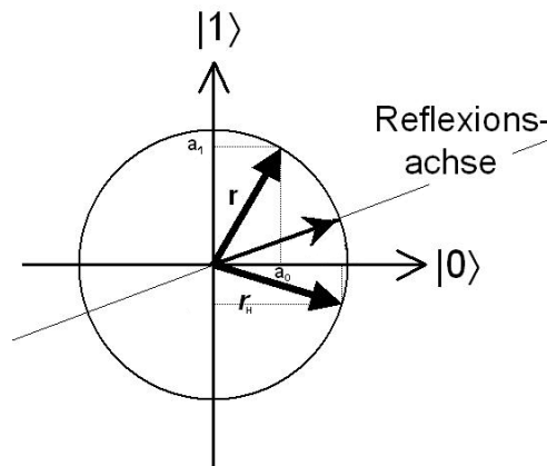
Abb.2: Graphische Veranschaulichung der Hadamard-Transformation
