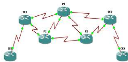
Gambar 1. Desain topologi jaringan VOIP berbasis MPLS VPN
