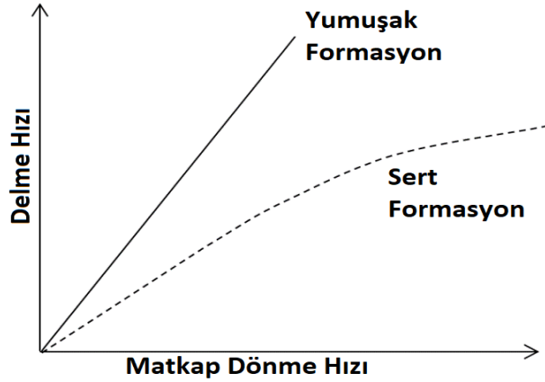
Şekil 1. Matkap dönme hızı ile delme hızı arasındaki ilişki Figure 1. Relationship between drill rotation speed and drilling speed
