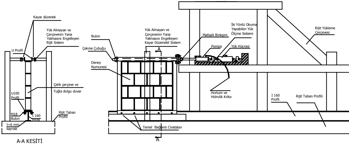
Şekil 1. Deneşlerde kullanılan yükleme sistemi (Korkmaz, 2004). Figure 1. The loading system used in the tests (Korkmaz, 2004).
