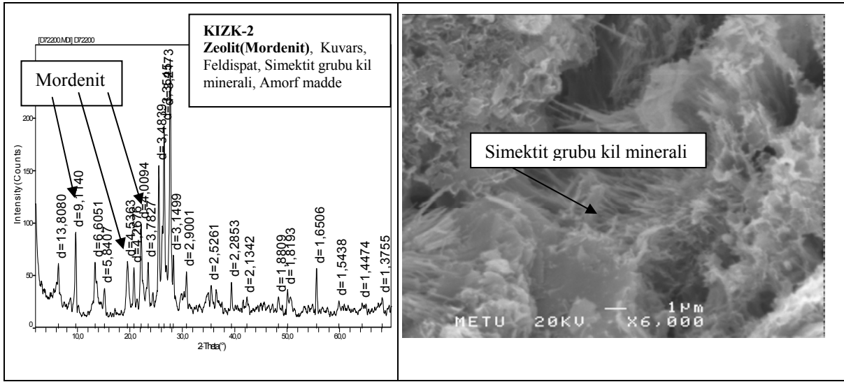
Şekil 7. KIZK-2 nolu Kayaç Örneğine ait X-Ray Difraktogram ve SEM mikrofrafı. Figure 7. X-Ray Diffractogram and SEM Micrograph of the Sample, numbered KIZK-2.
