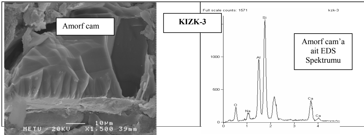
Şekil 8. KIZK-3 nolu Kayaç Örneğine ait EDS Spektrumu ve SEM mikrofrafı. Figure 8. SEM Micrograph and EDS Spectrum of the Sample, numbered KIZK-3.
