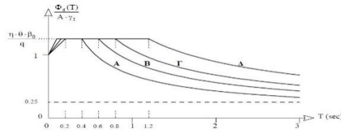
Şekil 2. Spektrum eğrisi (EAK2000)
