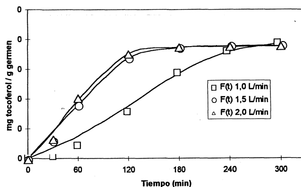
Figura 4 Efecto del caudal en el rendimiento de extracción de tocoferol
