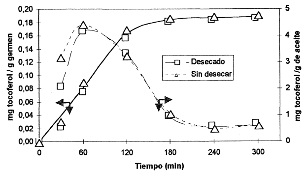
Figura 6 Efecto de la hidratación sobre el rendimiento de la extracción y la concentración de tocoferol en el aceite extraído
