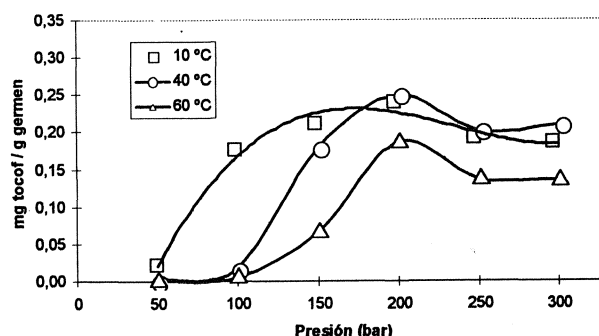
Figura 2 Efecto de la presión sobre el rendimiento de la extracción de tocoferol referida al trigo cargado
