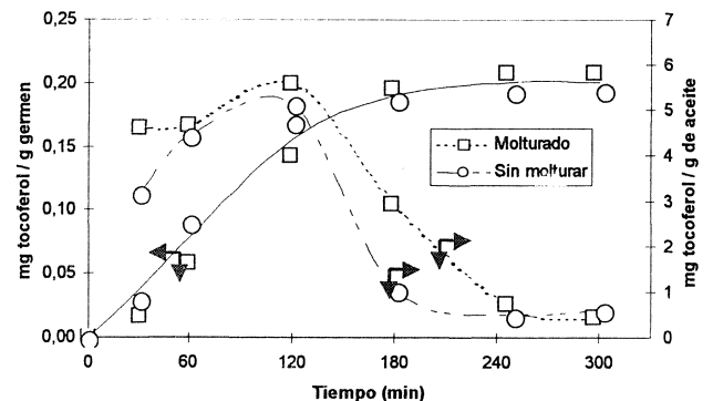
Figura 7 Efecto del diámetro de partícula sobre el rendimiento de la extracción y la concentración de tocoferol en el aceite extraído
