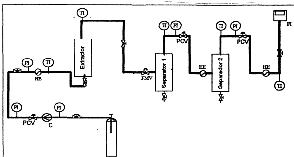
Figura 1 Diagrama de la planta de extracción con fluidos supercríticos
