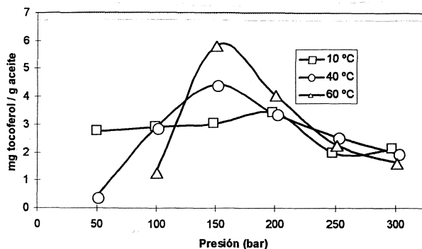
Figura 3 Efecto de la presión sobre la concentración de tocoferol en el aceite extraído
