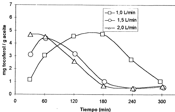
Figura 5 Efecto del caudal sobre la concentración de tocoferol en el aceite extraído
