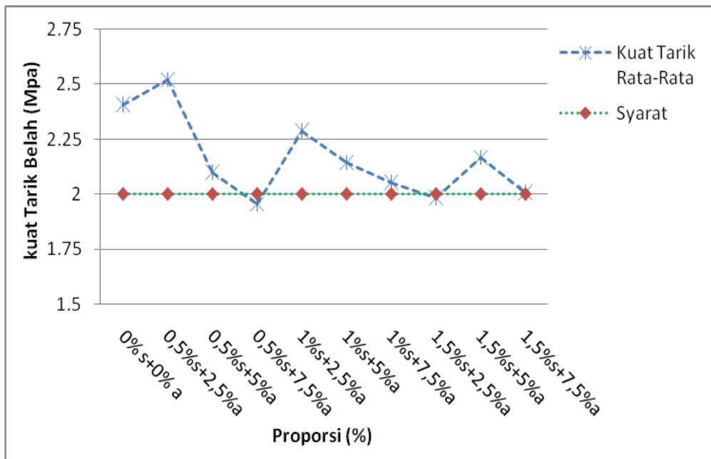
Gambar 4.9 Hasil evaluasi Pengujian Kuat Tarik Belah Beton Umur 28 Hari
