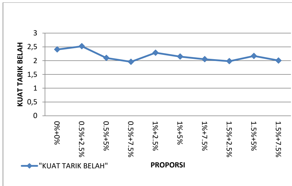
Gambar 2. Hubungan Penambahan Serat dari Sabut kelapa Terhadap Nilai Kuat Tarik Belah Beton
