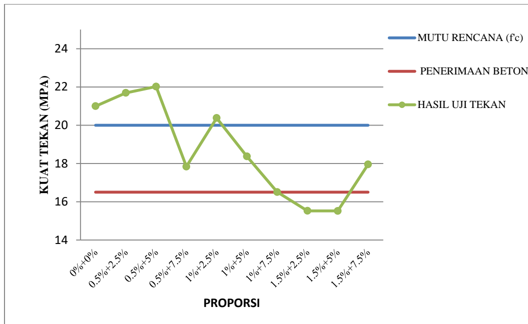
Gambar 4.7 Hasil Evaluasi Pengujian Kuat Tekan Beton Umur 28 Hari
