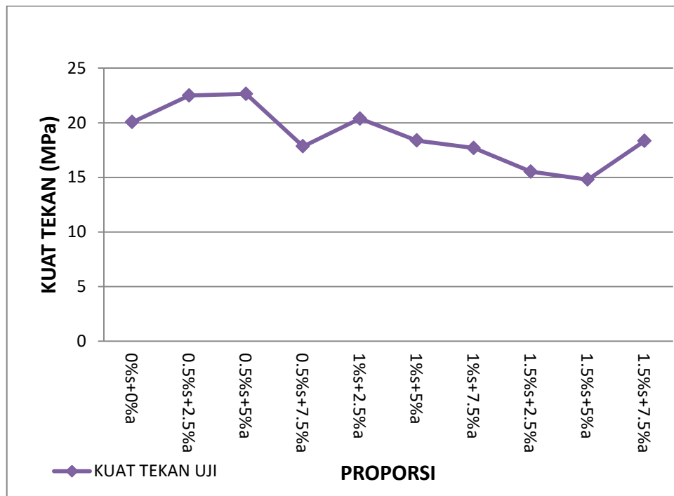
Gambar 1. Hubungan Penambahan Serat Terhadap Nilai Kuat Tekan Beton
