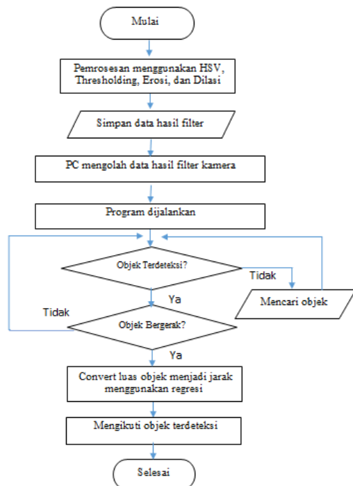
Gambar 4 Flowchart Sistem Perangkat Lunak
