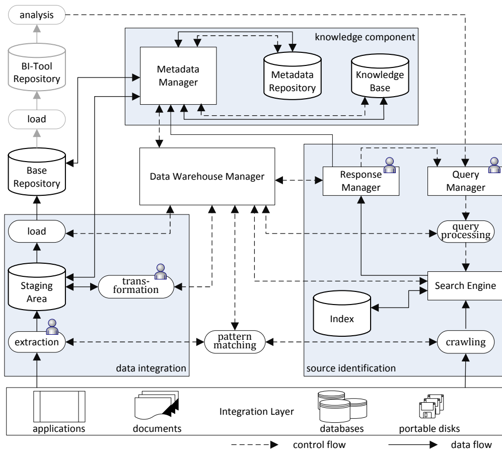
Abbildung 5: Architektur für den flexiblen ETL-Prozess
