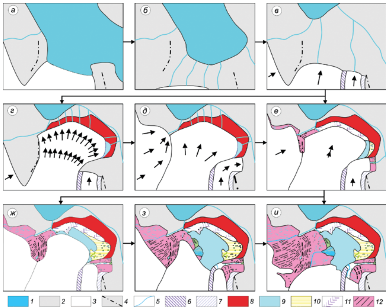
Рис. 3. Реконструкция динамики ледника Грёнфорд [22]:
