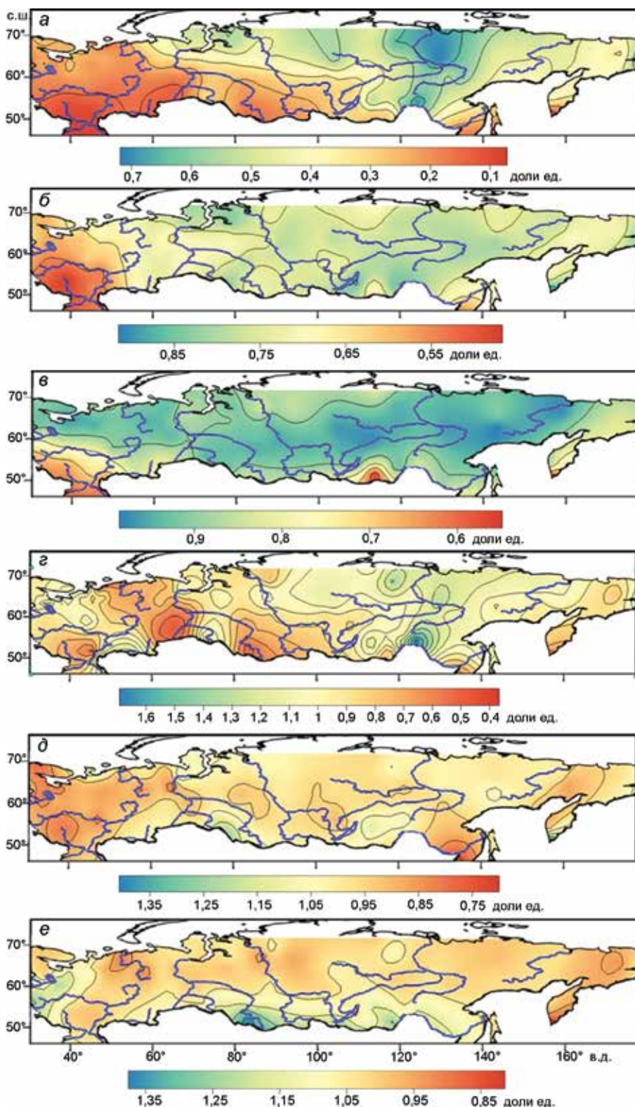
Рис. 3. Динамика толщины снежного покрова и её изменчивость.
