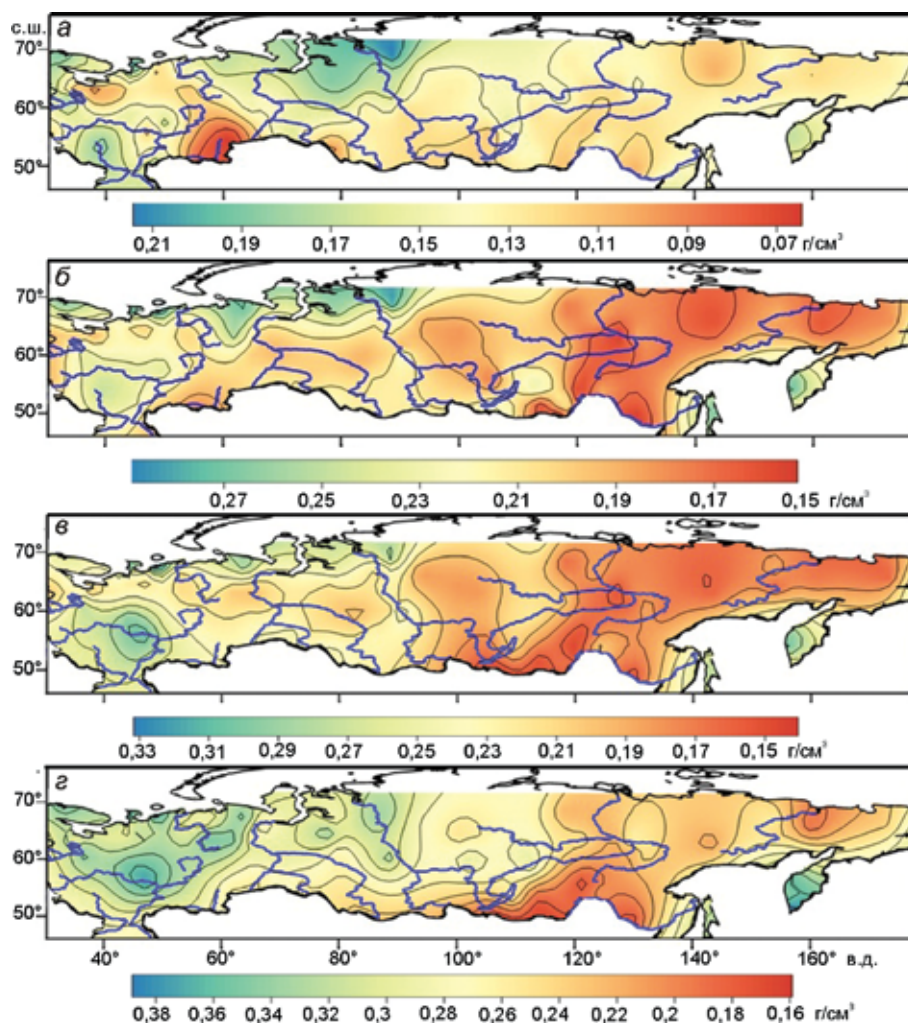
Рис. 4, а–з. Пространственная и временная изменчивость плотности снежного покрова на территории России. Средние значения плотности снежного покрова в период 2001–2010 гг.: а – ноябрь; б – январь; в – март; з – максимальные значения; изменение плотности снежного покрова в период 2001–2010 гг. относительно периода 1966–2000 гг.: д – ноябрь; е – январь; ж – март; жс – март; з – максимальные значения
