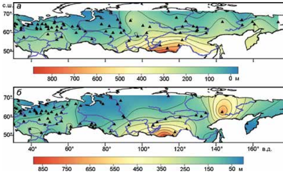
Рис. 1. Места расположения метеостанций с маршрутными снегосъёмками в лесу (а) и поле (б) и их высота над уровнем моря Fig. 1. The locations of the weather stations with measurements of snow cover depth on routes in the forest (а) and in the field (б) and their altitude above sea level
