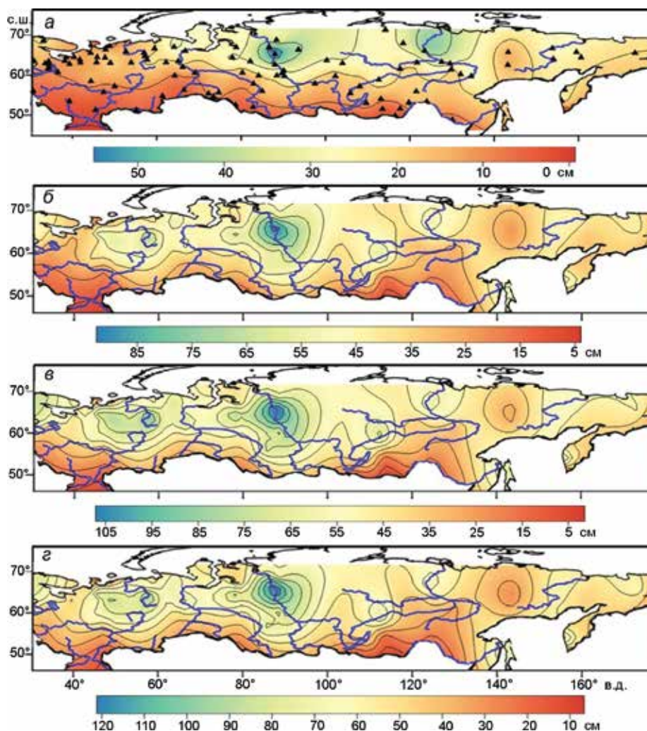
Рис. 2, а–з. Пространственная и временная изменчивость толщины снежного покрова на территории России. Средние значения толщины снежного покрова в 2001–2010 гг.: а – ноябрь; б – январь; в – март; г – максимальные значения; изменение толщины снежного покрова в 2001–2010 гг. относительно 1966–2000 гг.: д – ноябрь; е – январь; ж – март; з – максимальные значения; треугольник – места расположения метеостанций с данными маршрутных снегосъёмки толщины снежного покрова (а)
