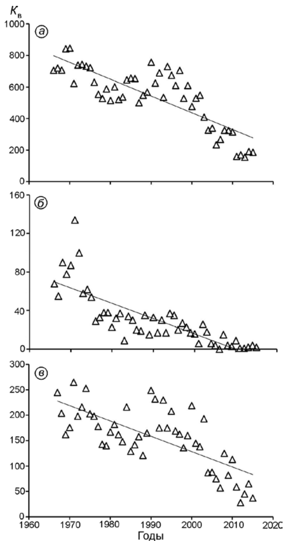
Рис. 3. Число сроков наблюдений K_b на метеостанции № 23405 (Усть-Цильма, Европейская часть России) за скоростью ветра за год (а, б) и календарную зиму (в) при скоростях ветра 6–10 м/с (а, в) и более 10 м/с (б) за период с 1966 по 2015 г.
