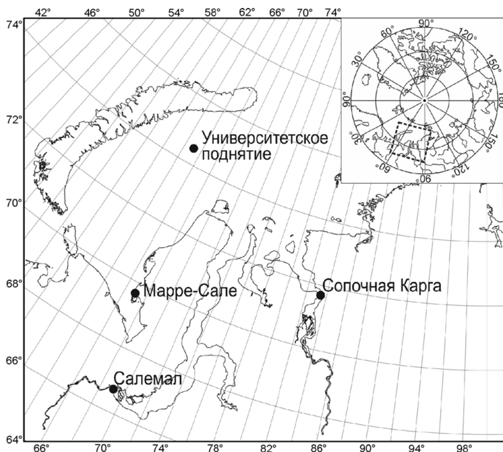
Рис. 1. Схема расположения участков, для которых проведено изучение метана в подземных льдах и мёрзлых отложениях
