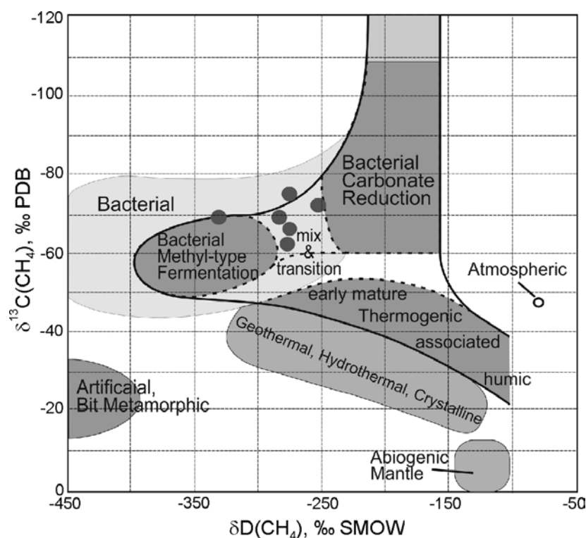
Рис. 4. Значения изотопного состава метана (чёрные точки), содержащегося в воздушных пузырьках пластовых льдов на CD-диаграмме Витикара [42] для классификации бактериального и термогенного природного газа в зависимости от соотношения изотопов \delta^{13}\text{C} (метана) и D (метана)
