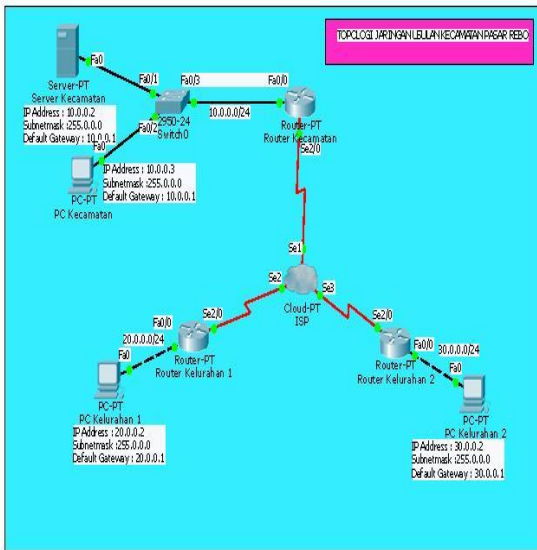
Sumber: Hasil penelitian (2013) Gambar 4. Topologi Jaringan VPN Kantor Kecamatan Pasar Rebo
