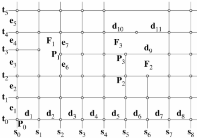
Рис. 1. Контрольна сітка для T-сплайнів
