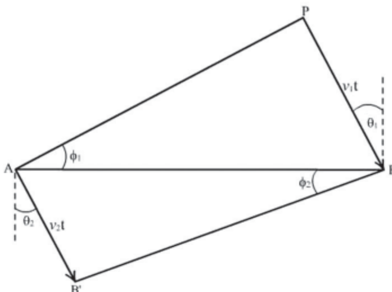
Figura 2. Una porción de onda incidente en un medio de índice de refracción n_1 , representada por el frente de onda AP penetra a un medio de índice de refracción n_2 . El frente de onda transmitido está representado por el frente de onda BB'. Mientras el extremo P del frente de onda incidente recorre una distancia v_1 t , el extremo A del frente de onda transmitido recorre una distancia v_2 t .
