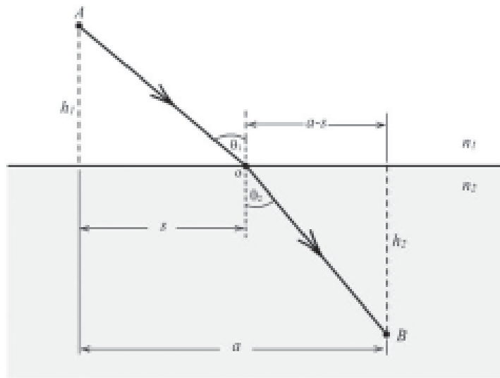
Figura 1. Un rayo de luz pasa del punto A del medio 1, índice de refracción n_1 , al punto B del medio 2, índice de refracción n_2 . La distancia horizontal entre los puntos A y B es a y la distancia vertical es h_1 + h_2 . Igualmente, la distancia horizontal entre el punto A y el punto de incidencia O es s .
