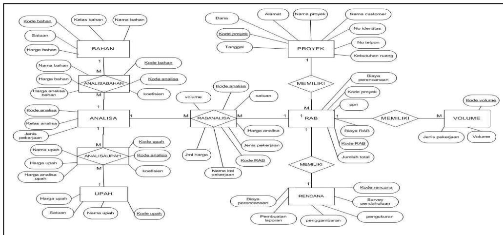
Gambar 5 ERD
