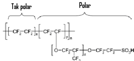
Gambar 1. Struktur Nafion.
