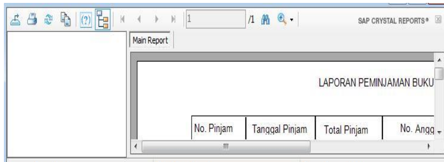
Gambar 20 : Form Laporan
