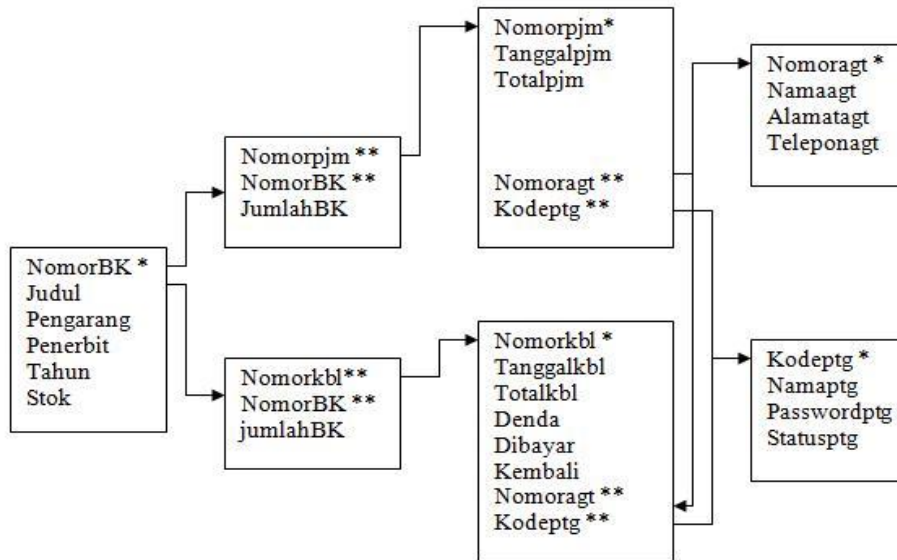
Gambar 1 : Normalisasi 3 dbperpustakaan
