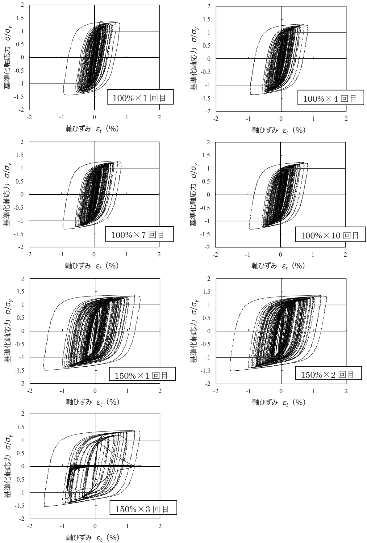
図 2.36 応力-ひずみ関係 (OSANS)
