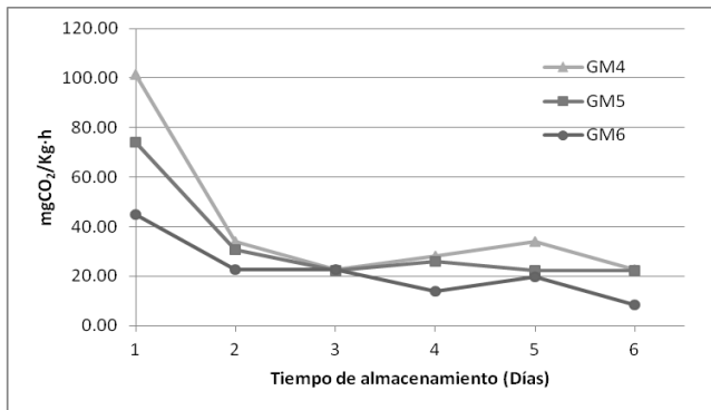
Figura 1. Intensidad respiratoria de frutos de mora de Castilla ( Rubus glaucus Benth) en tres estados de madurez durante almacenamiento refrigerado ( 2\text{ }^{\circ}\text{C} \pm 1\text{ }^{\circ}\text{C} ).
