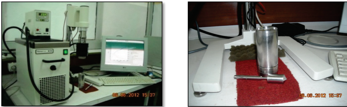
Figure 1 : Viscosimètre VT550.
