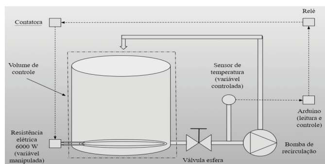
Figura 7: Disposição do sistema de medição e controle.
