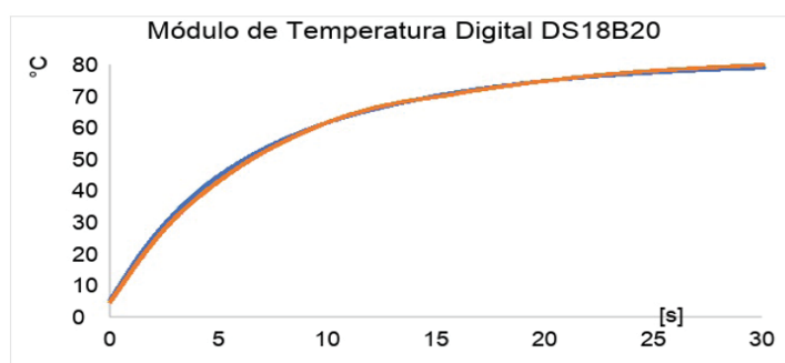
Figura 8: Curva de evolução do aumento de temperatura do sensor.
