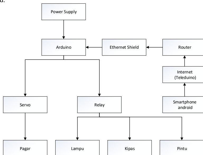
Gambar 4. Rancang Bangun Smarthome
