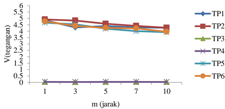
Gambar 6. Grafik Pengukuran pada Perintah Belok Kanan
