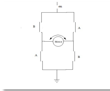
Gambar 8. Simulasi Prinsip Kerja H-Bridge
