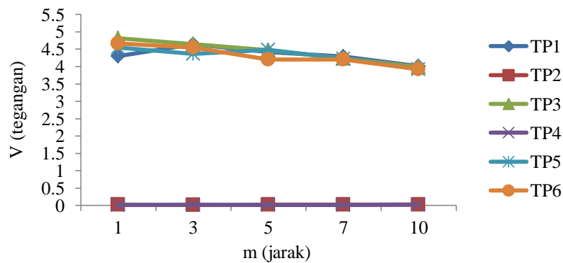
Gambar 5. Grafik Pengukuran pada Perintah Mundur
