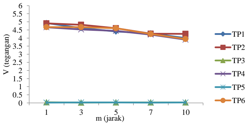
Gambar 4. Grafik Pengukuran pada Perintah Maju
