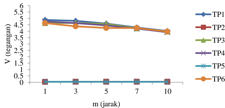
Gambar 7. Grafik Analisa Pengukuran pada Perintah Belok Kiri
