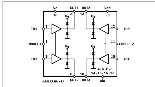
Gambar 1. Blok Diagram IC L293D
