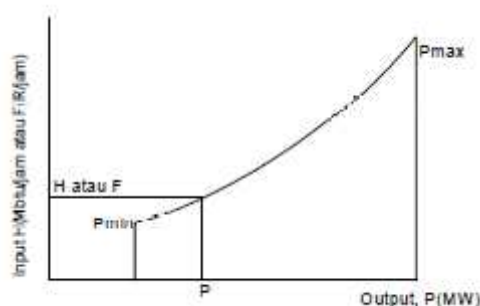
Gambar 1. Karakteristik input-output unit pembangkit termal (ideal)
