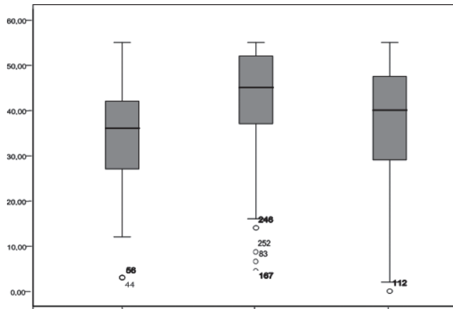
Figura 2. Diagrama de caja y bigotes para el puntaje total en AP según sexo.
