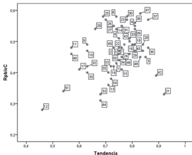
Figura 1. Distribución de la Tendencia correlacional de ítems arrojada por el análisis biserial puntual ( r_{bp} )
