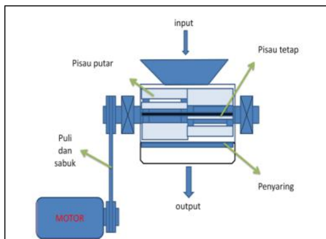
Gambar 2. Prototipe mesin pencacah sampah botol plastik
