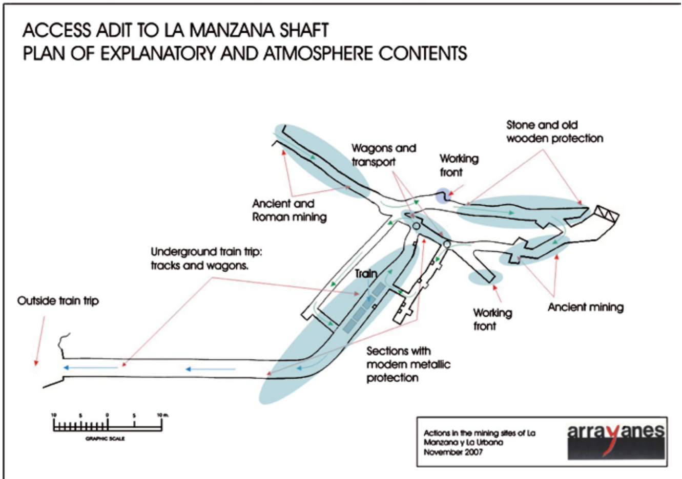
Fig. 14. Sketch of the project for the access adit of La Manzana (La Carolina) • Szkic projektu dostępu do sztolni kopalni La Manzana (La Carolina)
