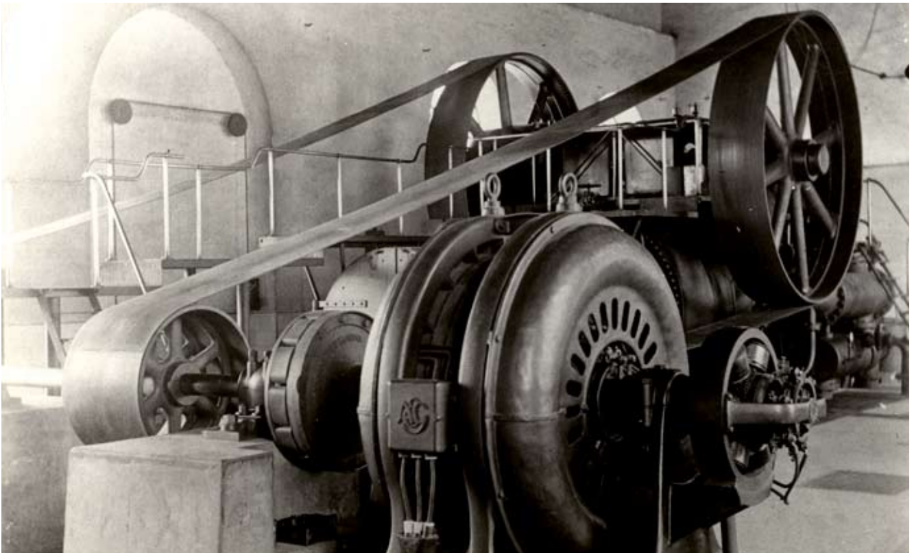
Fig. 9. Electric generator at the Electrical Central of La Manzana (La Carolina) • Generator w centrum energetycznym kopalni La Manzana (La Carolina)
