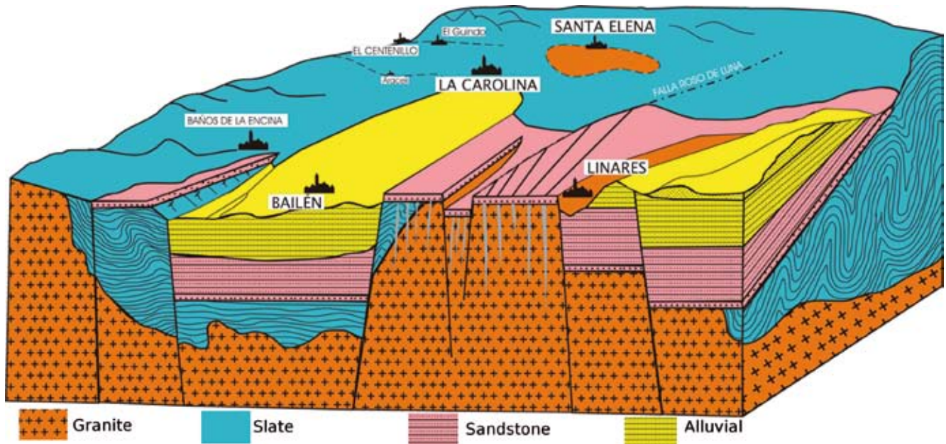
Fig. 3. Scheme of geological structure of the area Linares – La Carolina (after Azcárate, 1977, modified) • Schemat budowy geologicznej rejonu Linares-La Karolina (wg Azcárate, 1977, zmodyfikowany).
