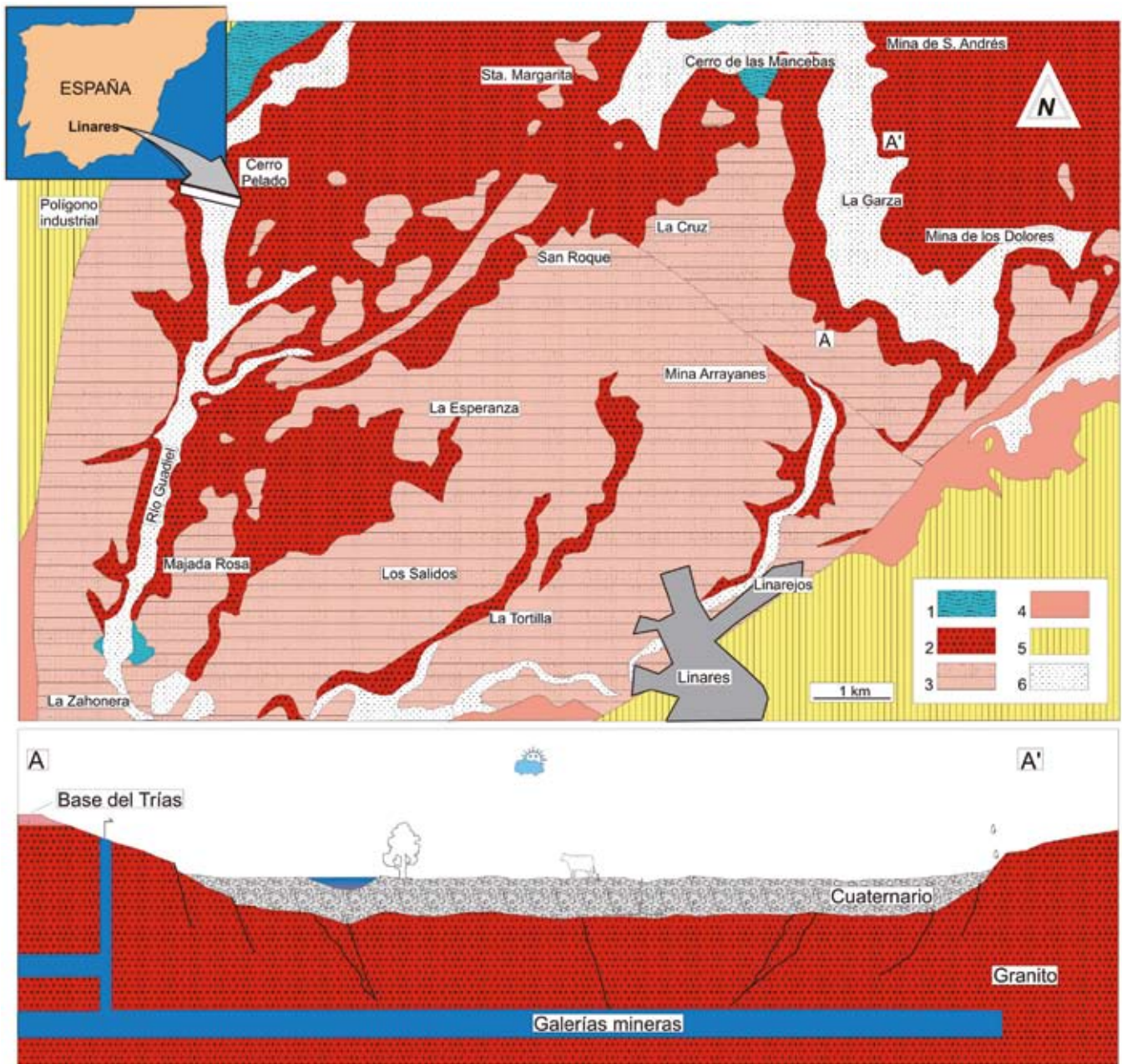
Fig. 4. Geological map of the southern area Linares – Cerro Pelado (after Dueñas et al. , 2000a). 1 – phyllites, 2 – granite, 3 – sandstone, 4 – clays, 5 – Triassic sediments, 6 – alluvial deposits • Mapa geologiczna obszaru południowego Linares-Cerro Pelado (wg Dueñas et al. , 2000a). 1 – fyllity, 2 – granit, 3 – piaskowce, 4 – gliny, 5 – osady triasu, 6 – osady aluwialne
