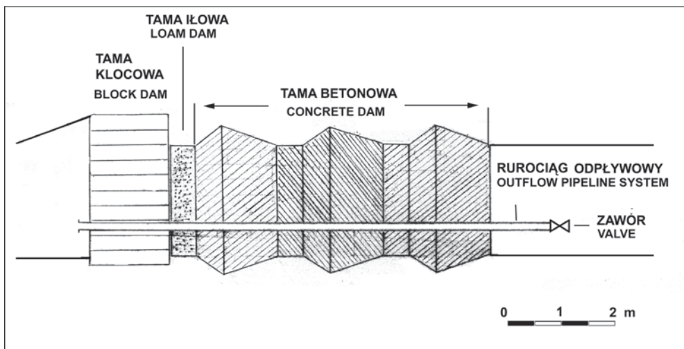
Fig. 5. Przekrój pionowy przez tamę wodną kłocowo-iłowo-betonową w chodniku Gussmann (poz. V)
