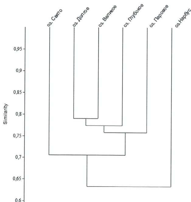
Рис. 3. Дендрограмма сходства флористического состава Пустынских озер
