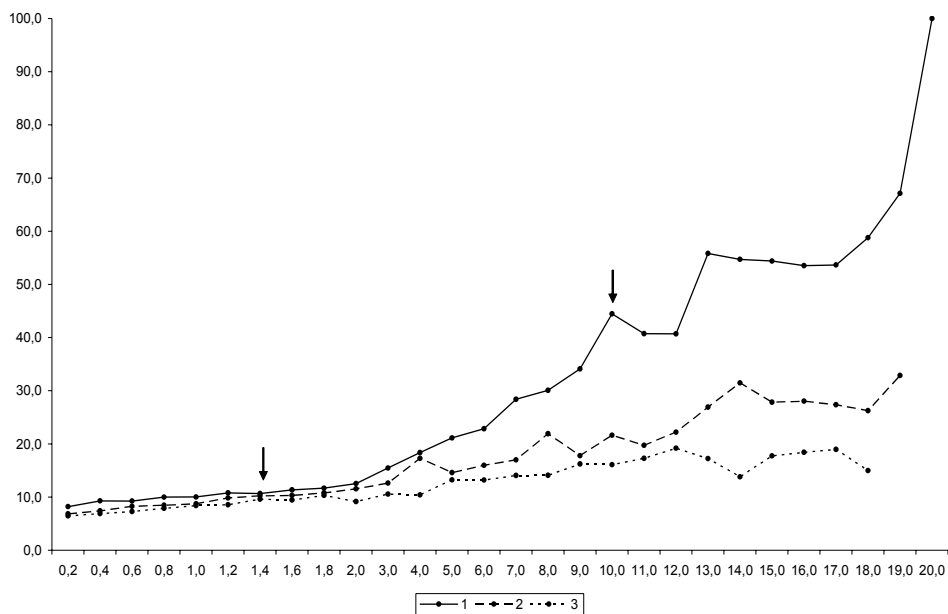
Рис. 1. Внесок до сумарної дисперсії трьох перших осей головних компонент залежно від розміру блоку для заплavnих колків: 1, 2, 3 – номери осей.
