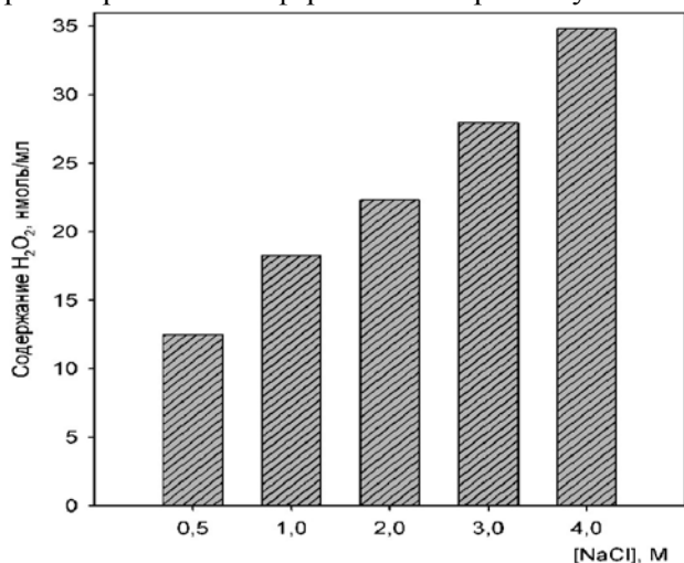
Рис. 2. Содержание H_2O_2 клеток D. salina , выращенных в условиях различной концентрации NaCl
