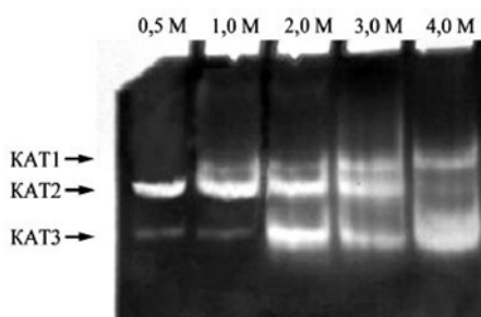
Рис. 4. Электрофоретические спектры каталазы клеток D. salina , выращенных в условиях различной концентрации NaCl
