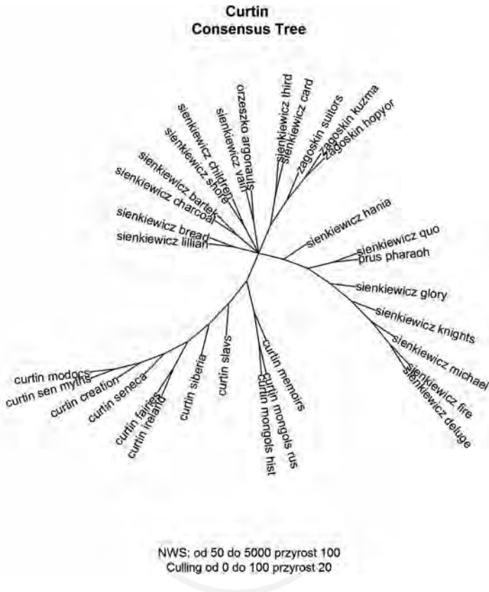
Wykres 1. Consensus tree dla wszystkich tekstów
