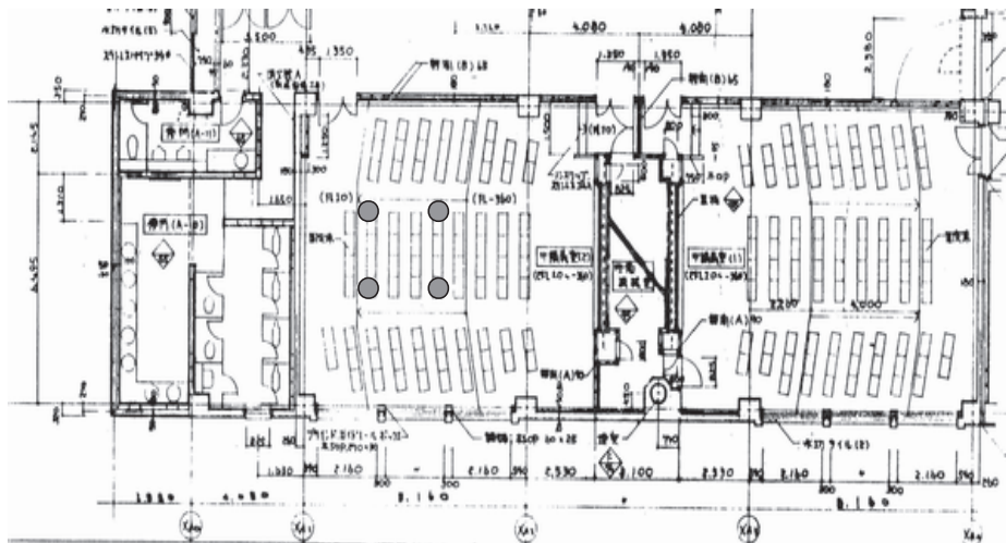
図2 平面詳細図と測定位置 ● 測定位置
