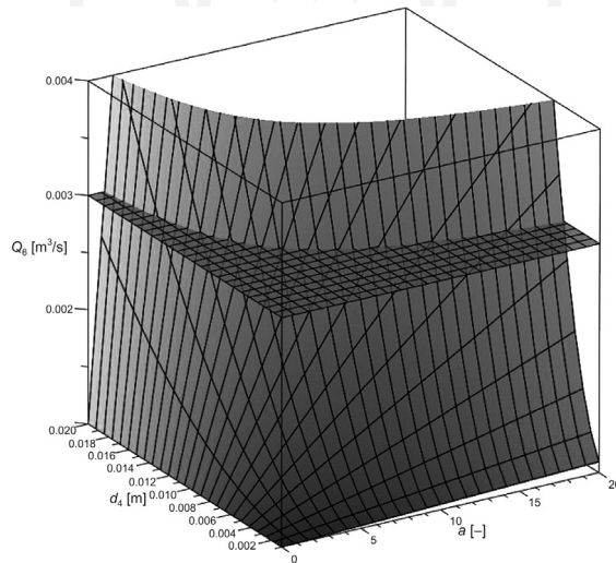
Fig. 4. The volumetric flow rate at the outlet Q_6 [m 3 /s] dependence of nozzle's number a [-] and nozzle's diameter d_4 [m] Rys. 4. Zależność objętościowego natężenia przepływu na wylocie Q_6 [m 3 /s] od ilości dysz a [-] oraz średnicy dyszy d_4 [m]
