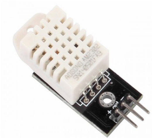
Figura 1. Sensor de Humedad y Temperatura del ambiente DHT22, tomado de tienda electrónica Robomart
