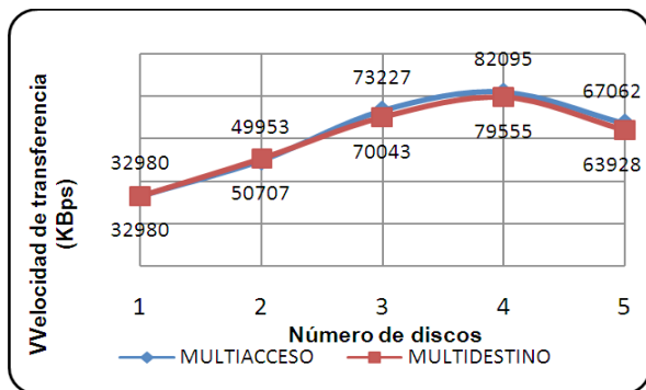
Fig. 3. Desempeño de los discos FC-SATA en las pruebas de múltiple acceso y múltiple destino en el servidor S7A
