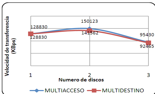
Fig. 4. Desempeño de los discos FC-SATA en las pruebas de múltiple acceso y múltiple destino en el servidor Power6.
