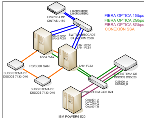
Fig. 1. Diagrama de la red de almacenamiento SAN.
