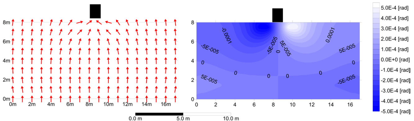
Figura 7. Rotaciones de Cosserat para el problema de valor de contorno
