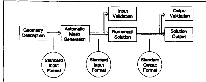
Figure 2: A modular numerical EM modeling code
