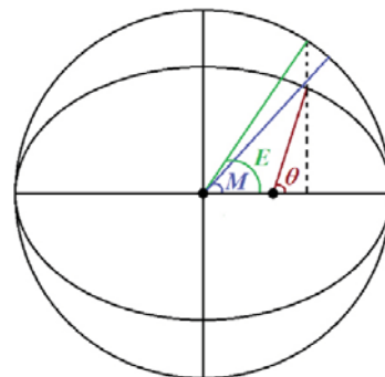
Fig. 9. Diagrama donde se ven los ángulos de la anomalía media M , anomalía excéntrica E y anomalía verdadera, la órbita y la circunferencia principal.
