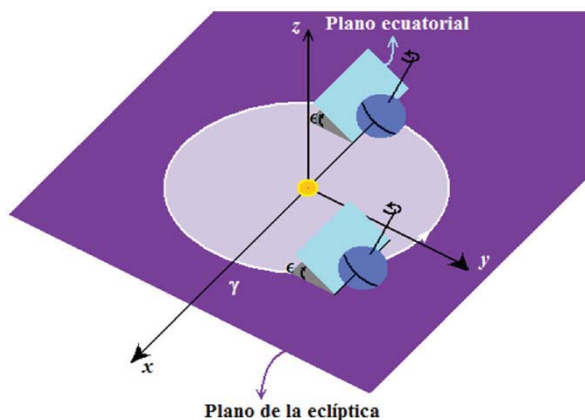
Fig. 5. Sistema de referencia cartesiano heliocéntrico eclíptico.
