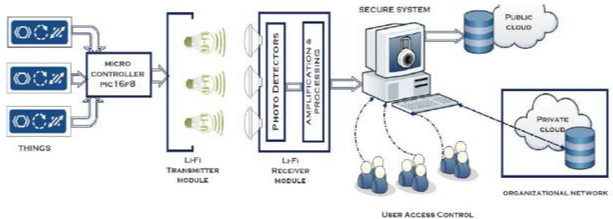
Figura 4. Sistema LiFi de apoyo de toma de decisiones en organizaciones [40].
